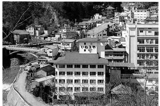
▲ こけしなどみやげ店もある土湯温泉
