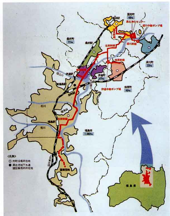
かんきょけいかくがいがようず 県北処理区管渠計画概要図
