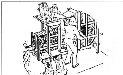
とうみ
