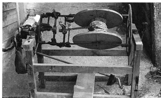
なわない機
