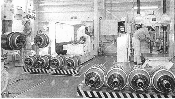
きかい工場〈モーターの組み立て〉
