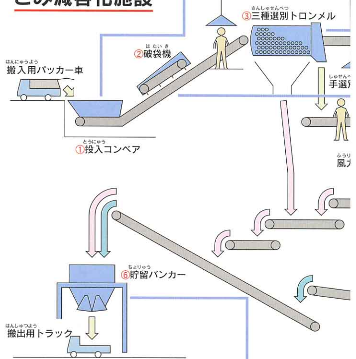
⑥ 貯留バンカー
