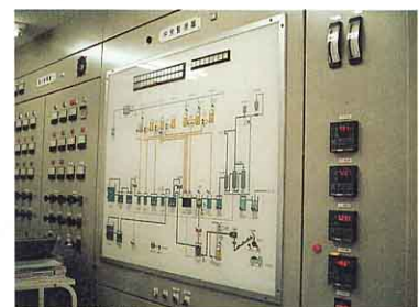
▲ 中央監視盤
