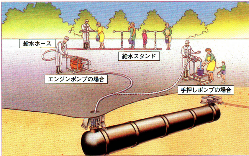
①耐震性貯水槽のしくみ
