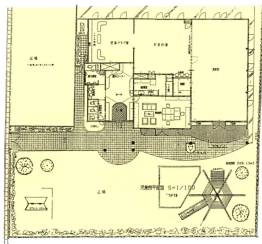
児童館平面図
