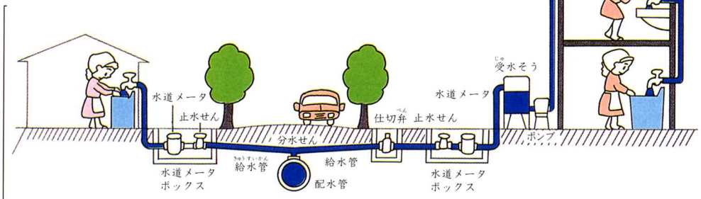
配水管から各家庭まで
