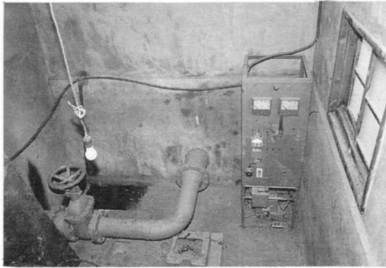
( 下川田揚水機場② )
