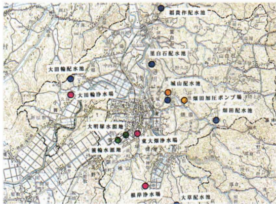
しせつ 浅川町水道施設配置図
