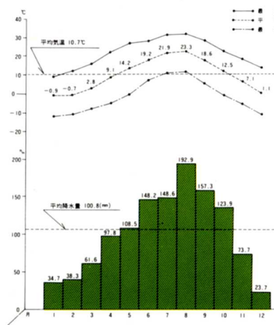
月別平均気温及び月別平均降水量 (1973年～1982年までの平均)
