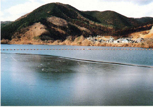
犬神ダム
