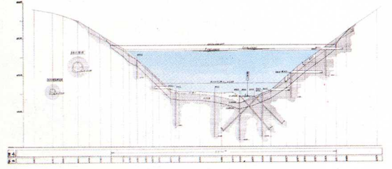
犬神ダムのだん面図①
