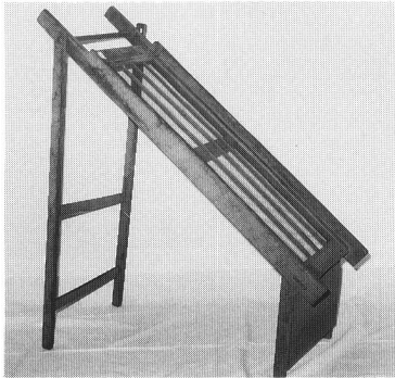
万石通
