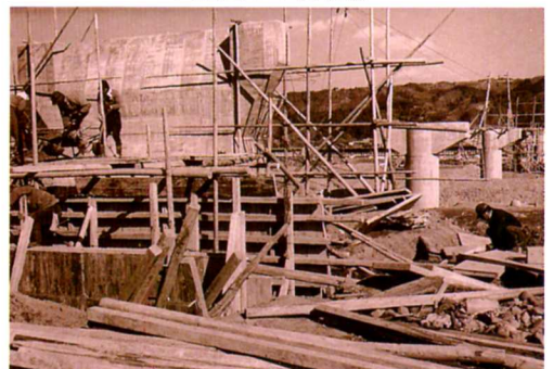
S35. 夢想橋改修
