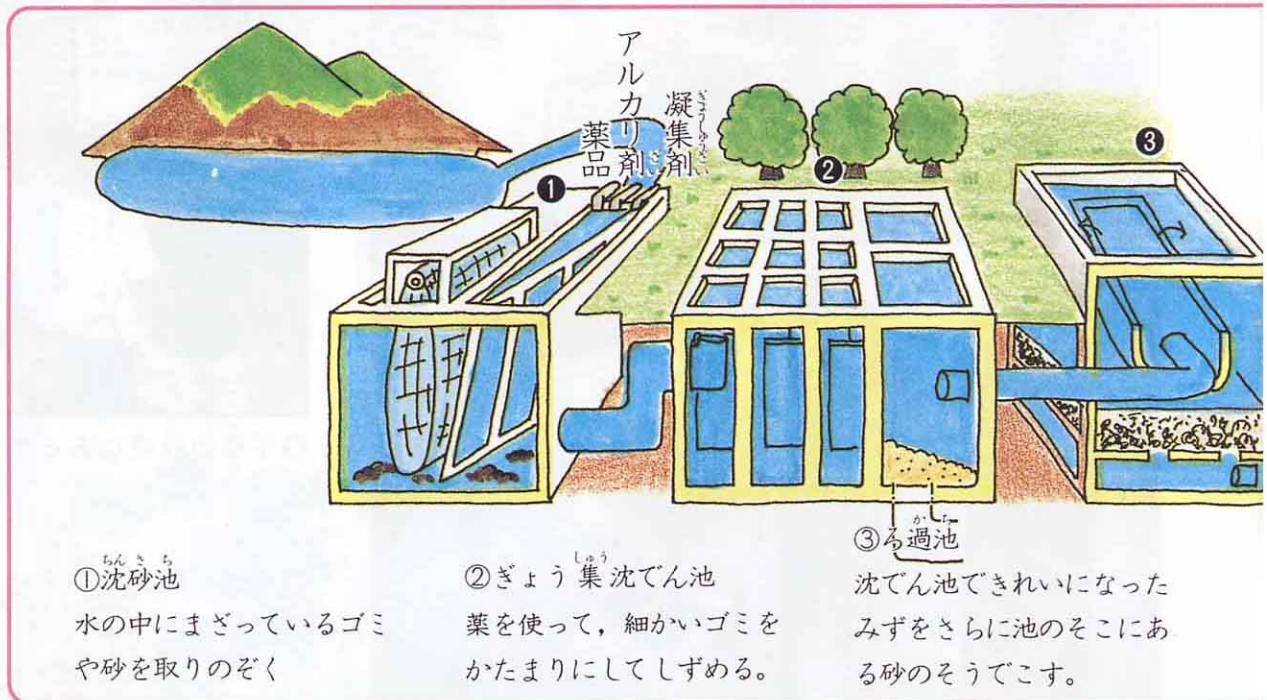
② じょう水場のしくみ (水道部パンフレット)
