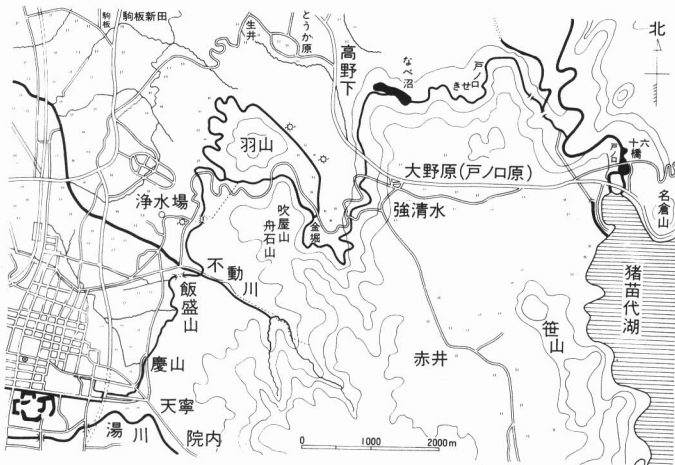
用水路完成図(猪苗代湖～若松)
