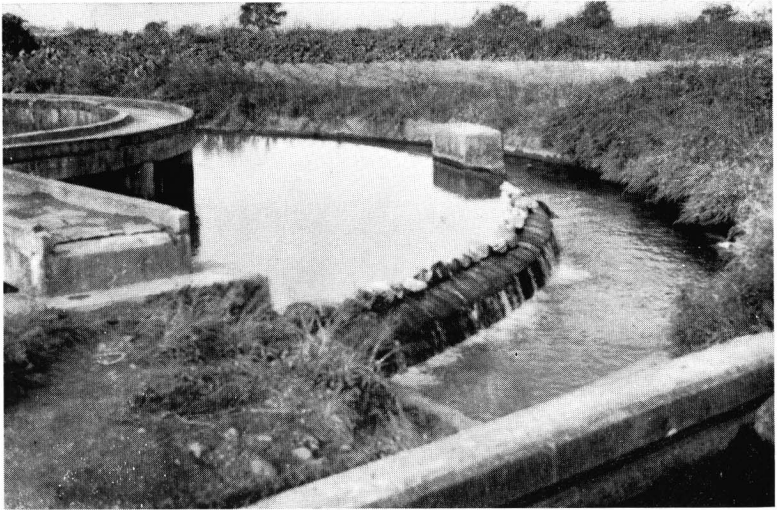
大川用水堰の円形分水装置（三重の円堤で調節する）
