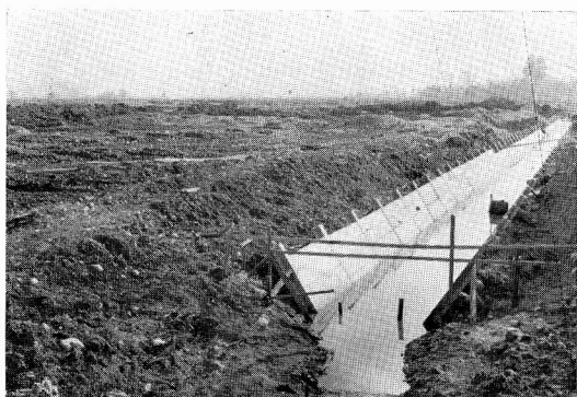
金屋付近の構造改善の用水路と整地
