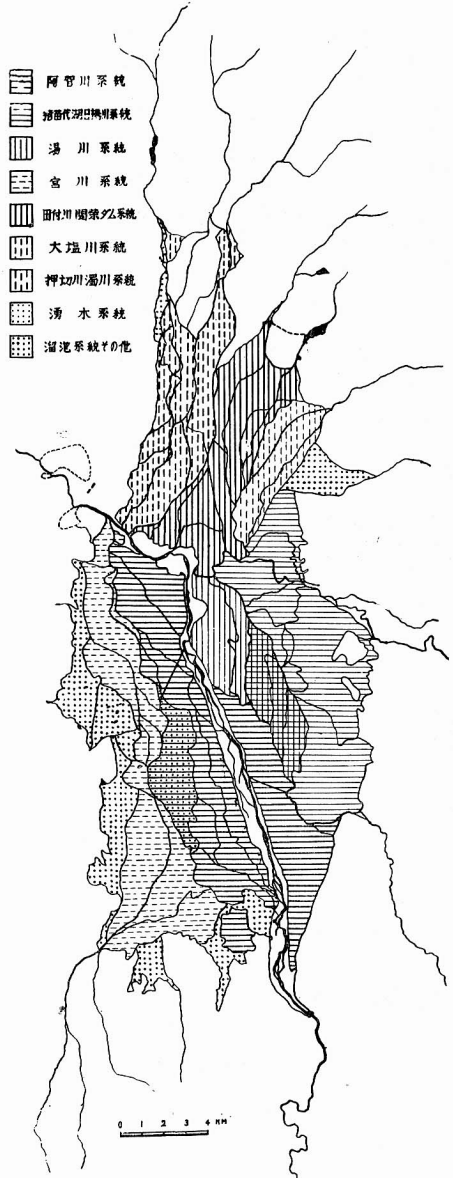
会津盆地灌漑用水系統図
