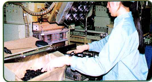
⑥ ゴムとリングをかたおしする
