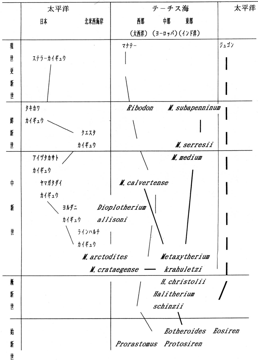
第12図 カイギュウ類の進化史 (a、b、c 図には現世・更新世のカイギュウ類を示す)
