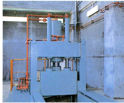
▲可燃性粗大ごみ破碎機 かねんせいそだい はさいき
