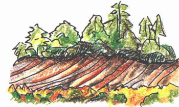
しゅう曲した地層
