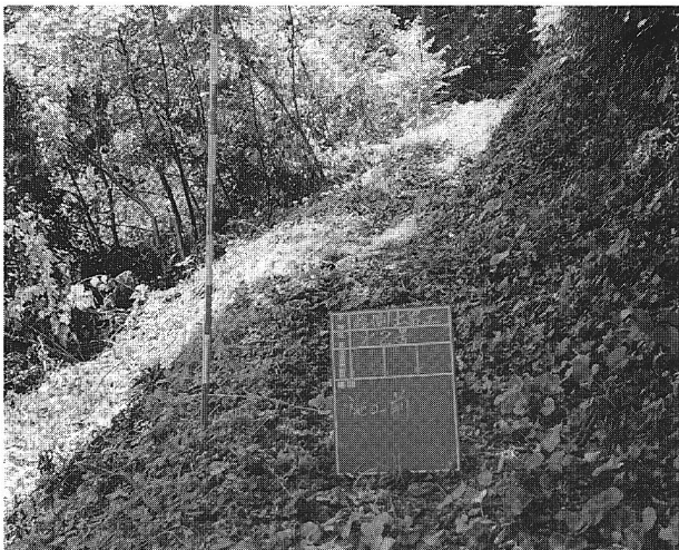
54 大内峠防護柵（施工前）図1
