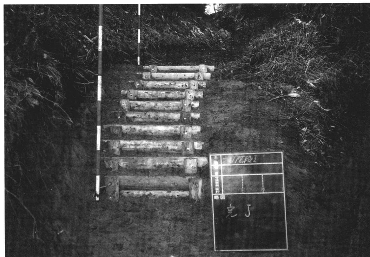
68 大内峠階段工 (施工後) 図2
