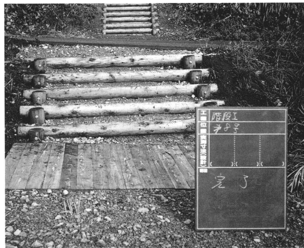
79 沼山峠階段工（施工後）図34-19
