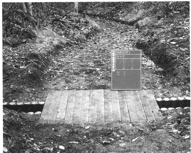
87 中山峠横断工（施工後）図34-17
