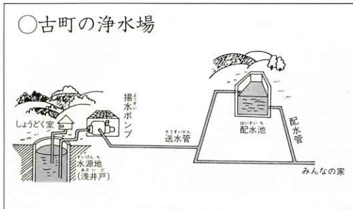
簡易水道のしくみ
