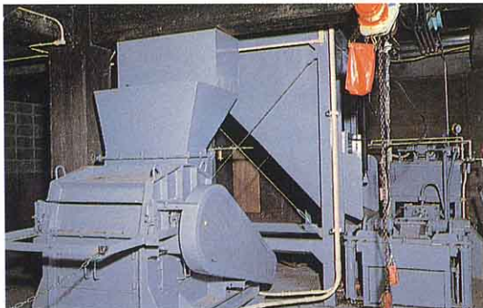
もえないごみをくだきプレスする機械
