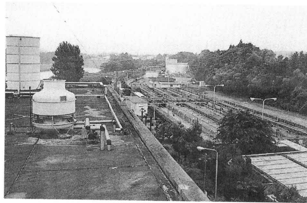
下水しより場
