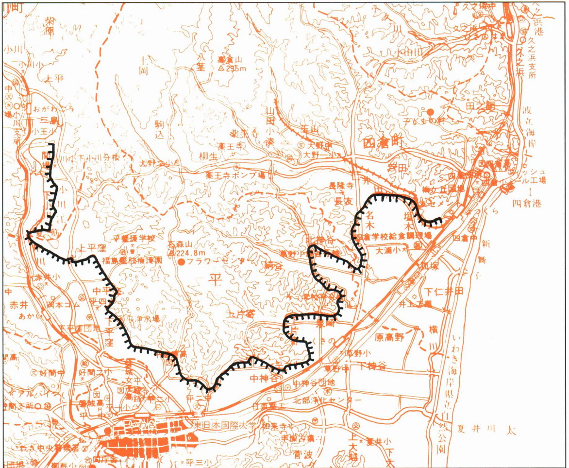
36-2 おがわえ 小川江すじの水路図
