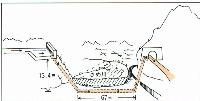
③ サイフオンのしくみ図
