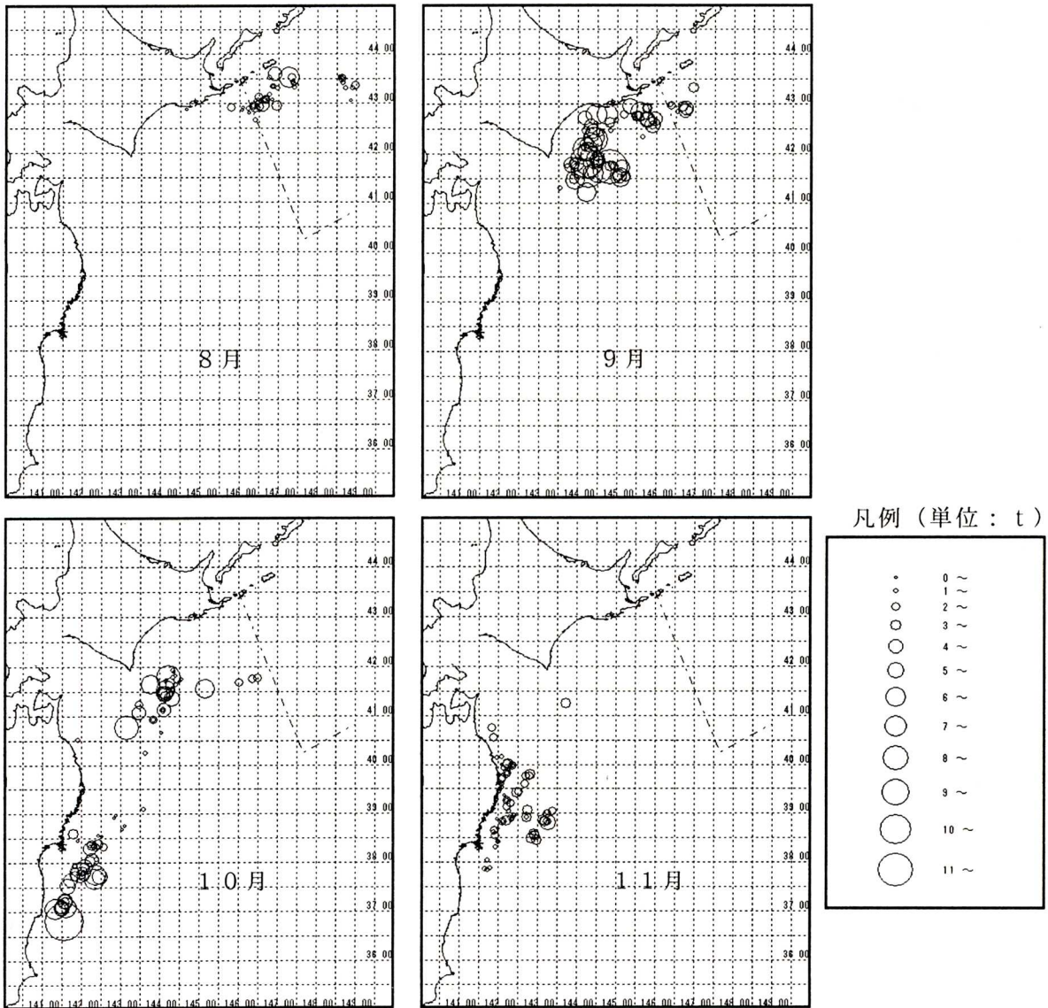
図4 平成13年漁期の月別サンマ漁場推移 (操業日別1網当たり漁獲量)
