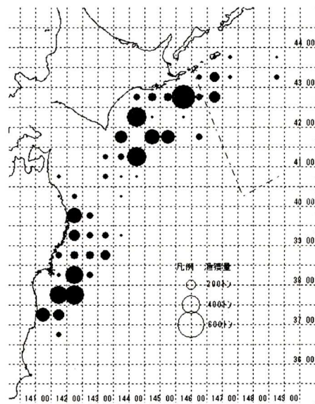
図6 平成13年度漁期漁獲量分布
