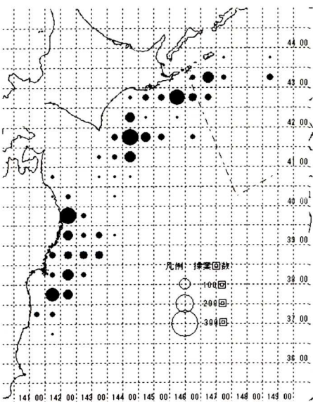
図5 平成13年漁期努力量分布
