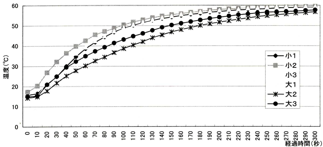
図2 60°C中でのホッキガイ中心温度の変化(サイズ別)
