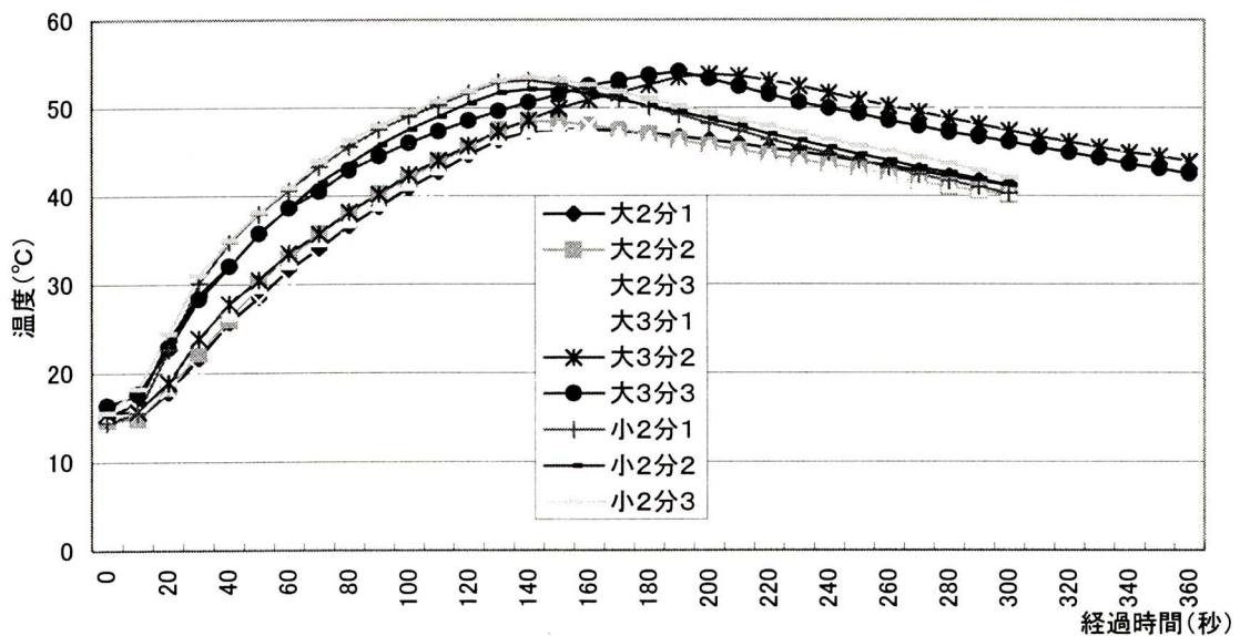
図3 60°C中で2分あるいは3分間加熱後放冷したホッキガイ中心温度の変化(大・小サイズ)
