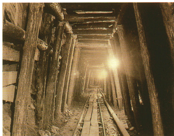
導水路トンネル（鮫川隧道）建設状況（昭和35年）
