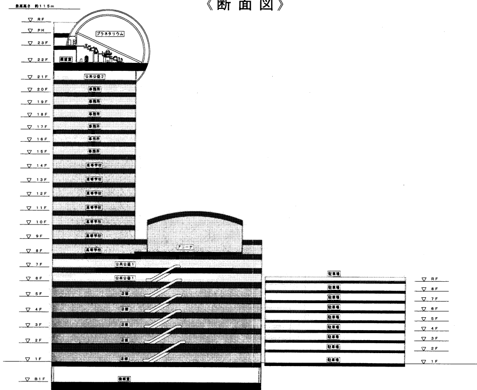
《断面図》
