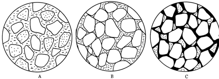
図-57 たい積岩のできかた
