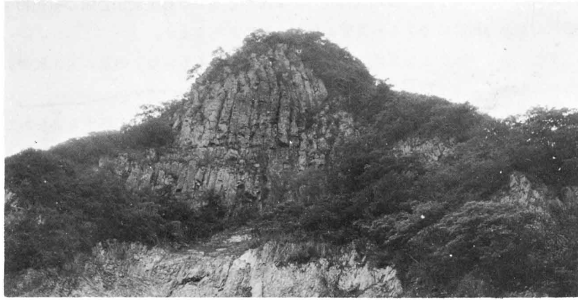
図-82 溶岩が流れずにかたまった山(会津若松・東山)
