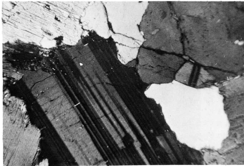
図-95 深成岩の顕微鏡写真(40倍)・・・(二本松)〈カコウ岩〉…等粒状組織 とうりゅうじょう
