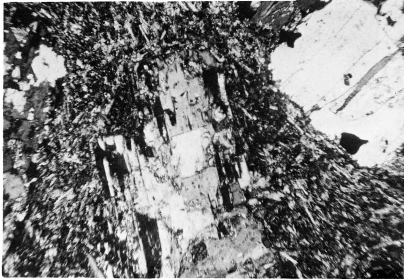
図-94 火山岩の顕微鏡写真(40倍)・・・(吾妻山)〈アンザン岩〉…斑状組織 はんじょう
