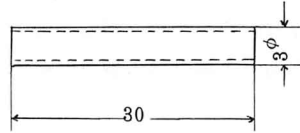
エ 回転軸(B)
