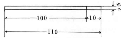
オ 固定心棒(B)
