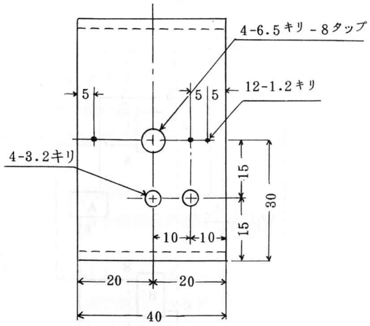
ウ 固定心棒
