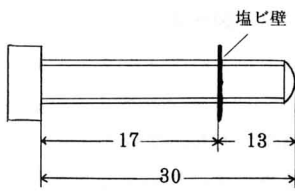
エ 木台
