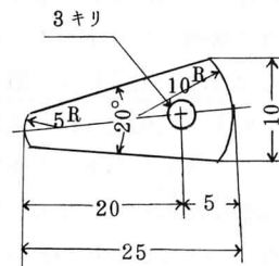
④ 接点
