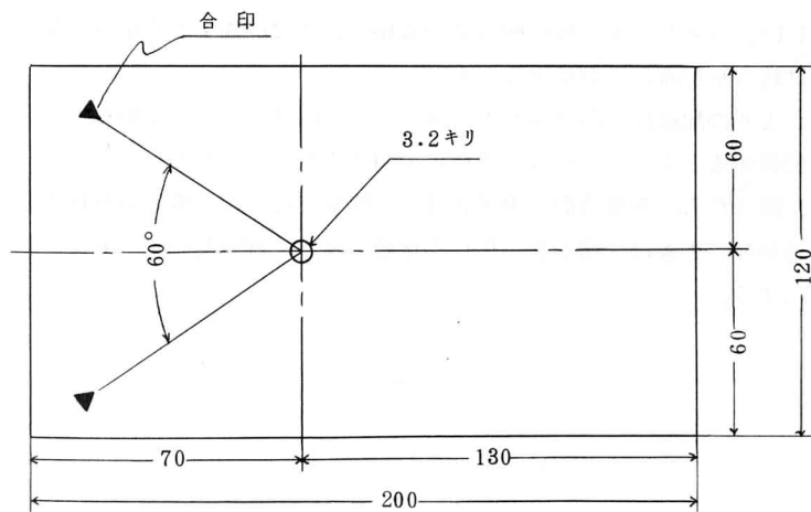
⑤ 木台
