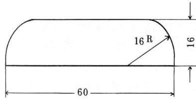
⑤ 木台
