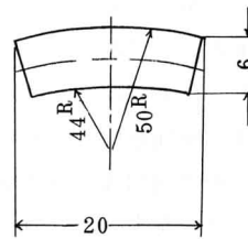
③ 接点板
