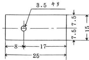
(4) 支持板
