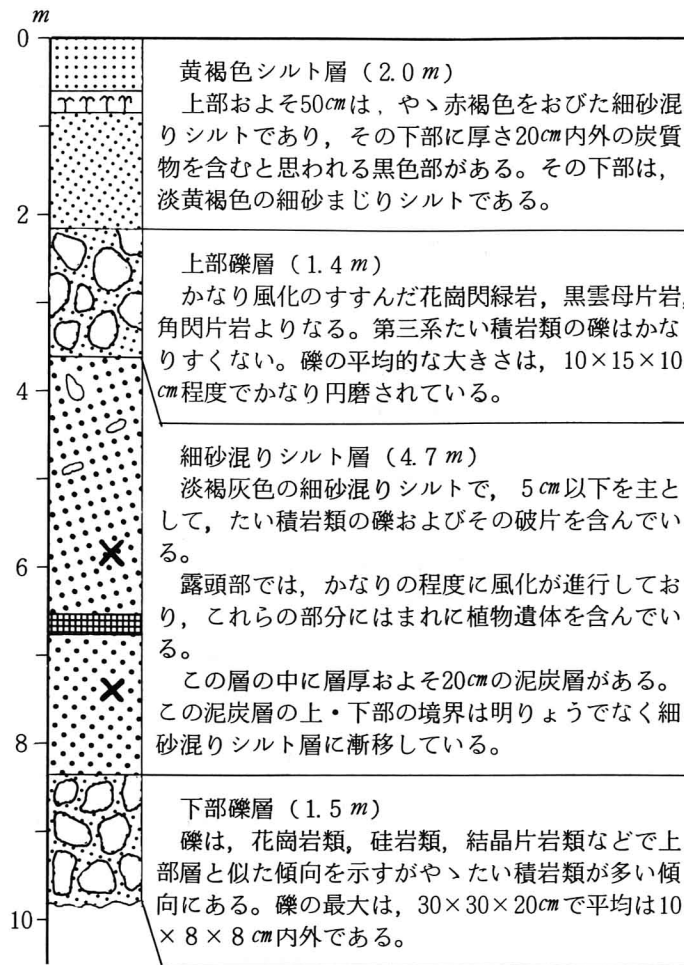
図2 段丘たい積物の例
