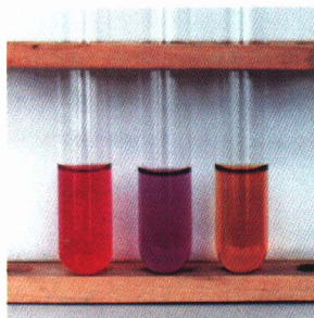
野ボタンの花 (酸性、中性、アルカリ性)
