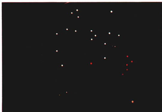
北天投影図
