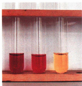
シソの葉 (酸性、中性、アルカリ性)
