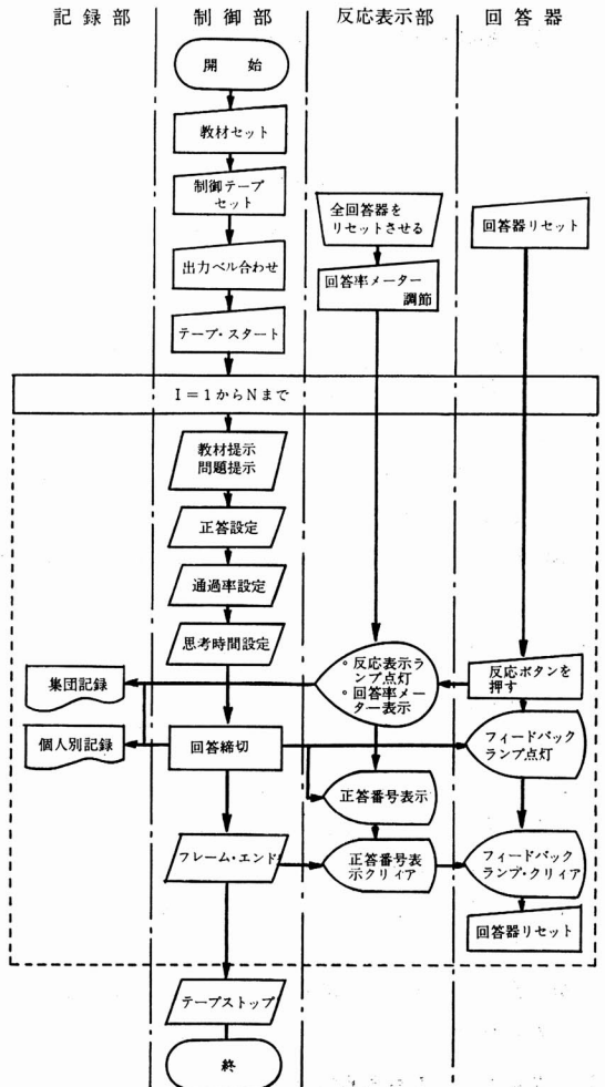
図 4 全自動進行のフローチャート
