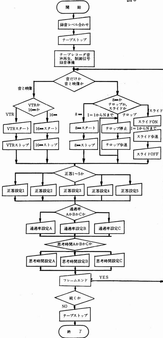
制御プログラム作成フローチャート
