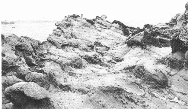
いわき波立海岸（波立薬師）
