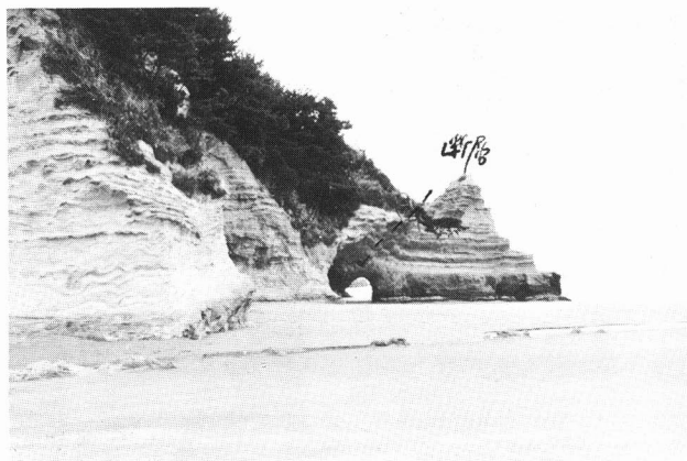
海食崖と海食洞（いわき豊間海水浴場）
