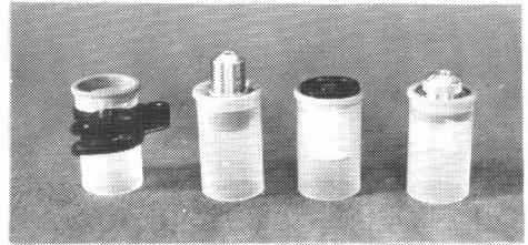
内筒（フィルムケース）に取りつけた各種レンズ 左から、ルーペ、対物レンズ、接眼レンズ、解剖顕微鏡レンズ
