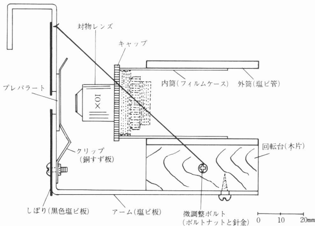
解剖顕微鏡レンズを取りつける場合
